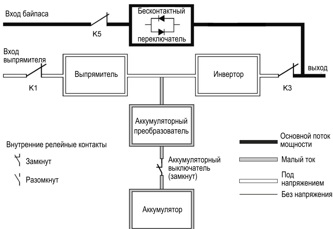
Рис. 2-4: Путь прохождения тока через ИБП в режиме энергосбережения
